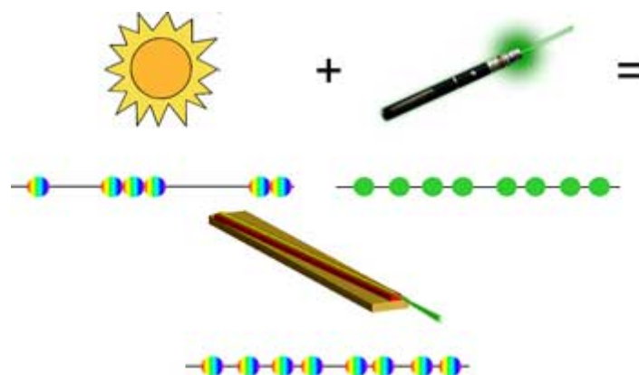
Abb.1: Die neuartigen Hybrid-Lichtzustände kombinieren die spektral breitbandigen Eigenschaften einer in erster Ordnung inkohärenten thermischen Quelle wie der Sonne mit den ko-
