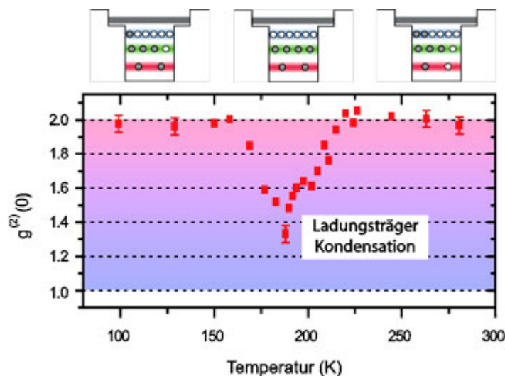
Abb.3: Im oberen Bildteil sind schematisch die Besetzungen der Quantenpunktzustände für drei verschiedene Temperaturen von 90, 190 und 290 K eingezeichnet (rot: Grundzustand, grün: erster, blau: zweiter angeregter Zustand; grau = besetzt, weiß = unbesetzt). Sie illustrieren die erhöhten stimulierten Emissionsanteile der bei 190 K erzeugten Hybrid-Lichtzustände aufgrund der erhöhten Besetzung des oberen angeregten quantisierten Zustandes. Trägt man den zentralen Intensitätskorrelationskoeffizienten g^{(2)}(\tau=0) als Funktion der Temperatur der Superlumineszenzdiode auf (unten), liegt er zwischen den Grenzen des thermisch inkohärenten und des in zweiter Ordnung kohärenten Lichtzustands. (TU Darmstadt)
